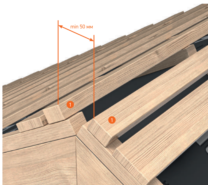
1. Подконьковая обрешетка
