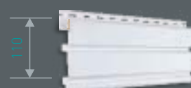
3 Добор [ 110 мм ] используется в Узле Наружный угол + Добор
