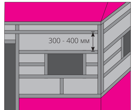
рис. 26 Горизонтальная обрешетка
