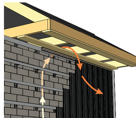
Рисунок 20. Кровельный свес
