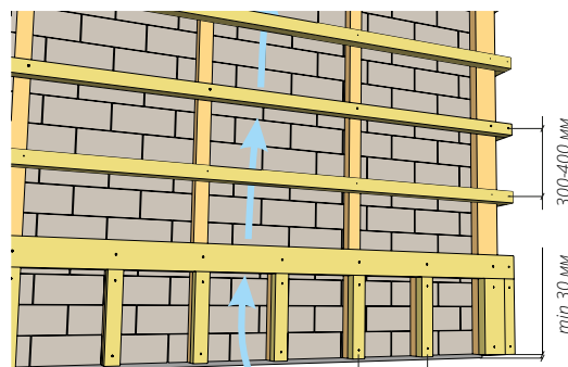
Рисунок 12. Деревянная обрешетка с цоколем
