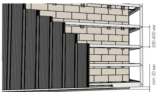
Рисунок 13. НФС без цоколя
