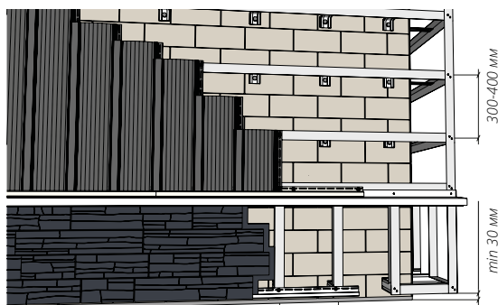
Рисунок 11. НФС с цоколем
