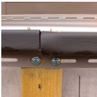
Неверное соединение J-профилей. Саморезы вкручены в края перфорации.
