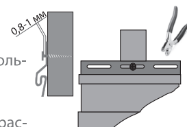
Ножницы по металлу
