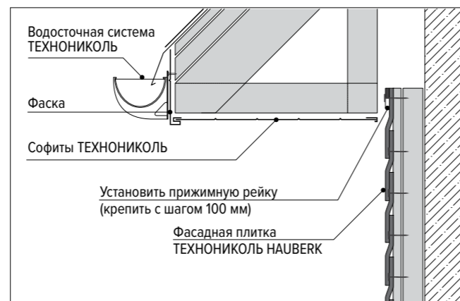
Рис. 23. Монтаж верхнего ряда под карнизным свесом. Вариант 1
