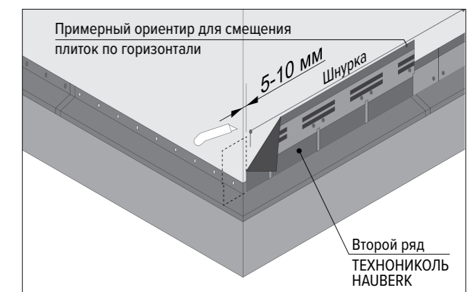
Рис. 8. Монтаж первого и последующих рядов фасадной плитки
