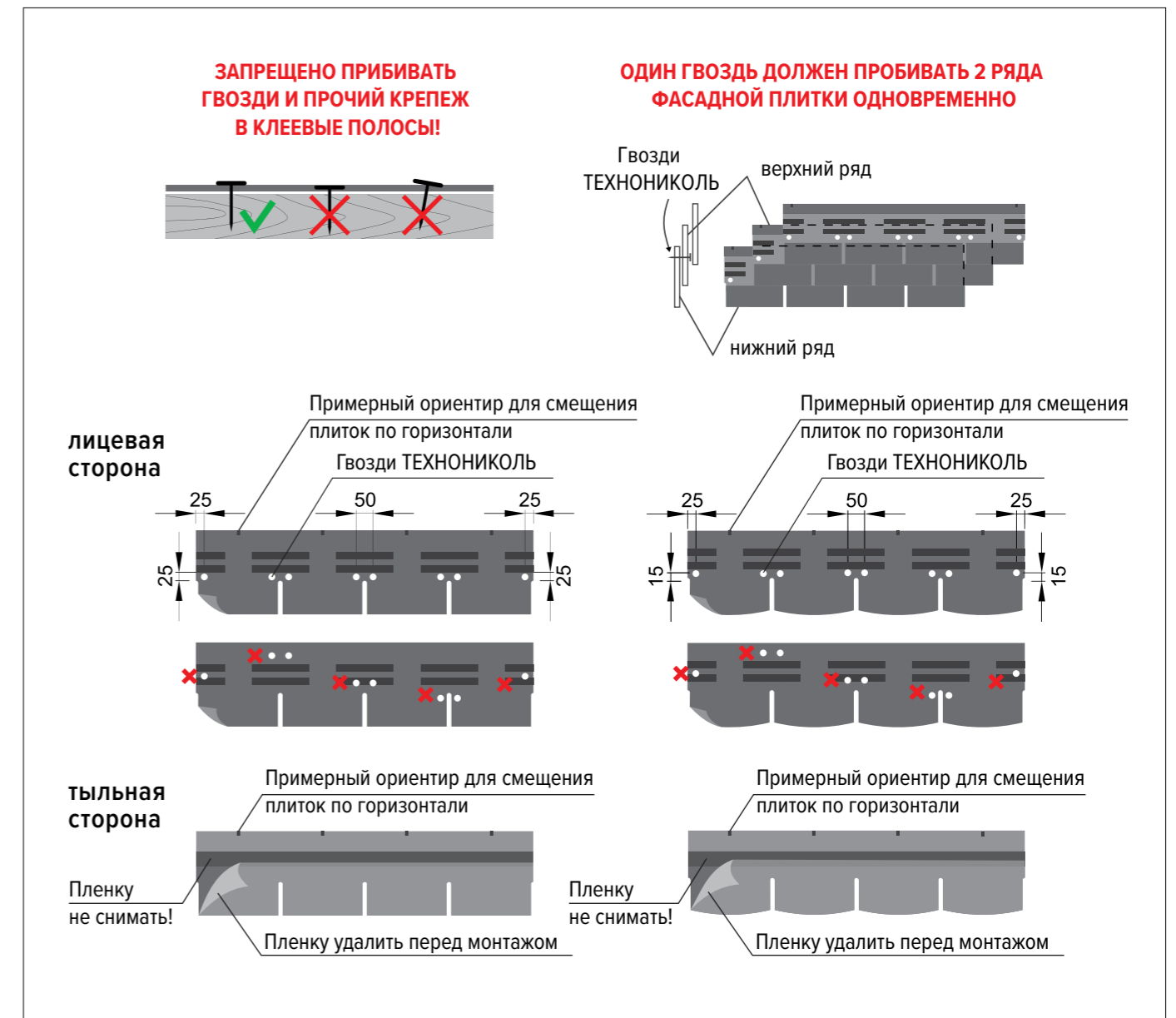
Рис. 2. Схема крепления фасадной плитки на 8 гвоздей
