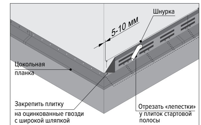
Рис. 7. Монтаж стартовой полосы фасадной плитки
