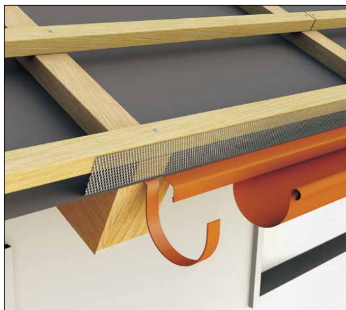
Вариант 2: Капельник заходит в водосток
