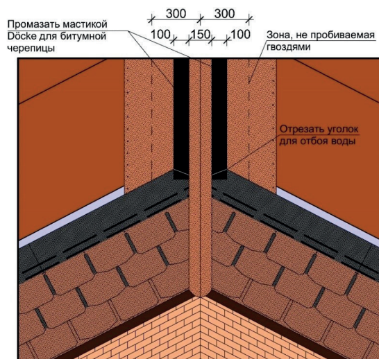
Рис. 26. Выполнение открытой ендовы.
