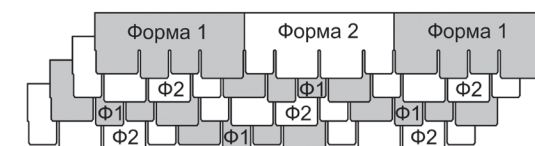
Рис. 20. Схема чередования гонтов гибкой черепицы Döcke LUX коллекции «Саппоро».
