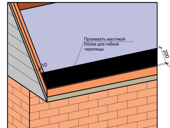
Рис. 21. Герметизация карнизного свеса под укладку ламинированной черепицы Döcke.
