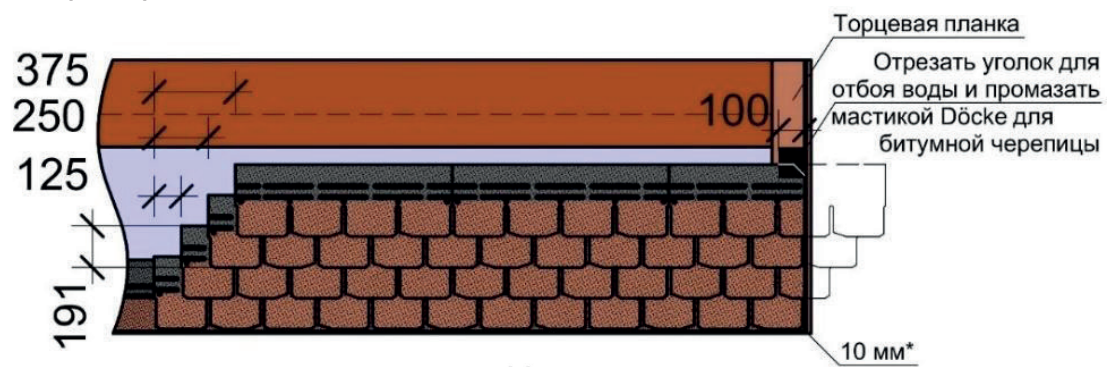
в - Форма нарезки «сланец»
