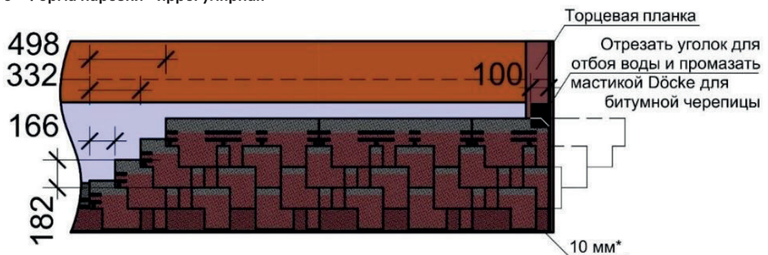
б - Форма нарезки «иррегулярная»
