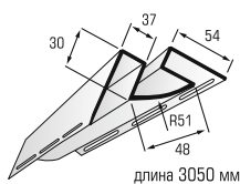
1 внутренний угол
