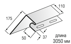
5 околонная планка
