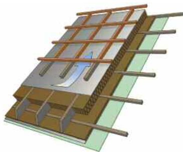
Рис. 8. Устройство дополнительного слоя теплоизоляции с внутренней стороны
